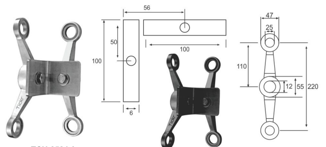
TCH-8524 A Four Way Spider without Fin (90°)
