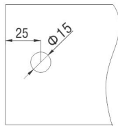
Size & Cutout Details for TCH-8438, TCH-8438 A & TCH-8438 R U Connector
