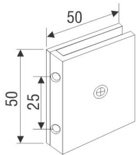
Size & Cutout Details for TCH-8438, TCH-8438 A & TCH-8438 R U Connector
