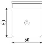
Size & Cutout Details for TCH-8442, TCH-8442 A & TCH-8442 R L Connector
