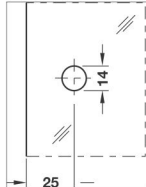
Size & Cutout Details for TCH-8442, TCH-8442 A & TCH-8442 R L Connector
