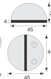
TCH-8404 Glass Door Stopper
