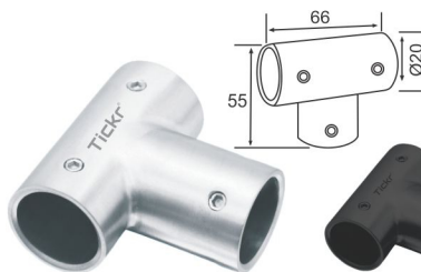
TCH-8459 Rod to Rod T Connector
