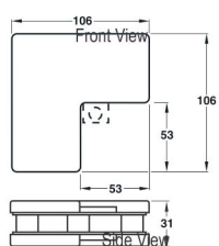
TCH-8408 Small L
